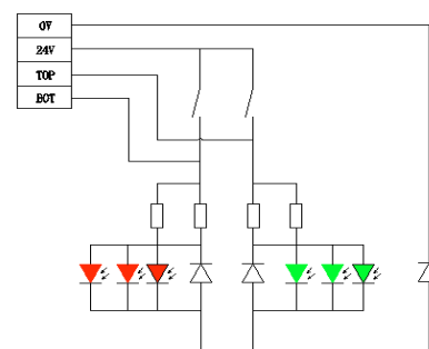
CONNESSIONI ELETTRICHE ELECTRICAL CONNECTION
